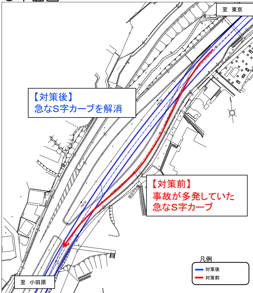
改良計画平面図
