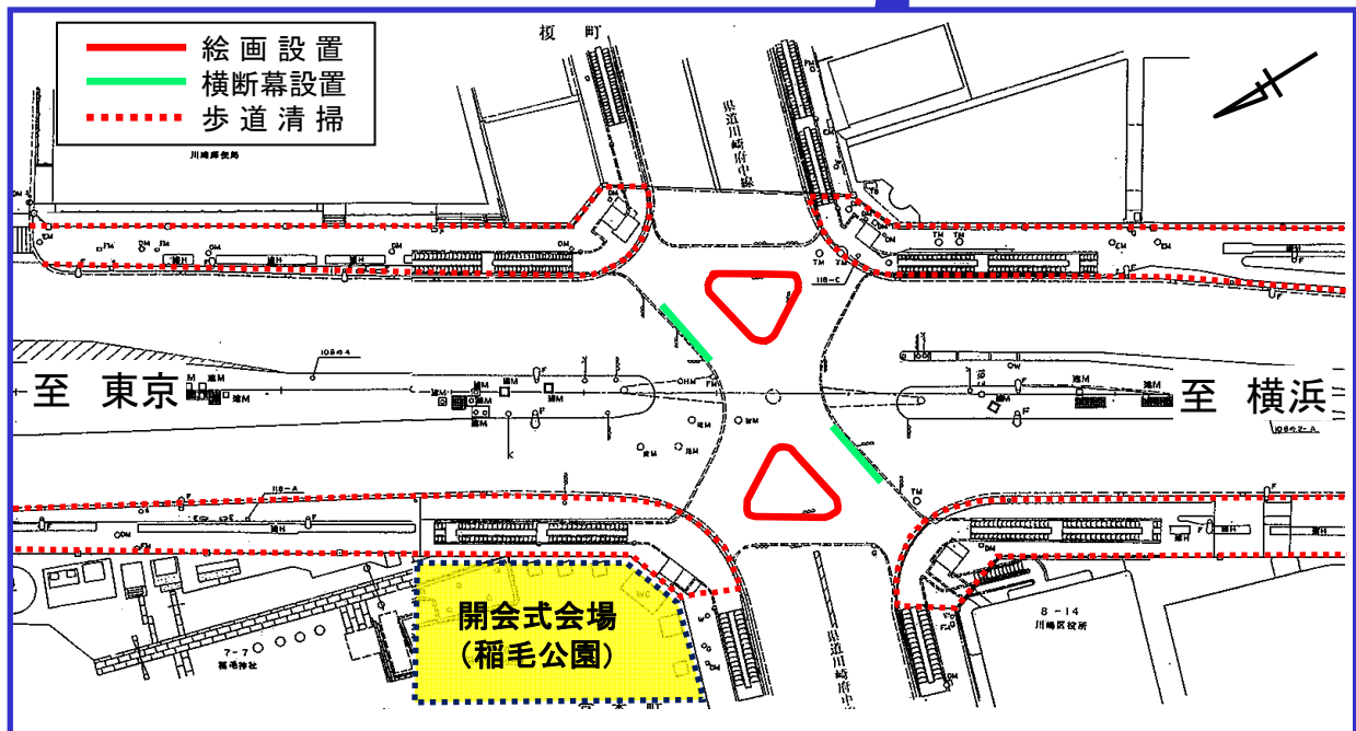
川崎ハローブリッジ付近 詳細図
