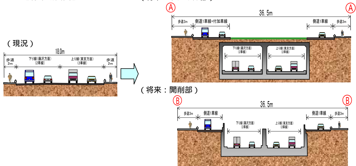
【標準断面図】
