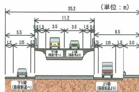
図 小田原箱根道路断面図① (立体部)
