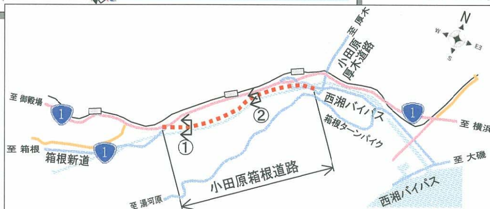
図 平面図
