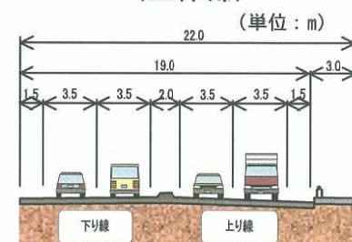
図 小田原箱根道路断面図② (一般部)
