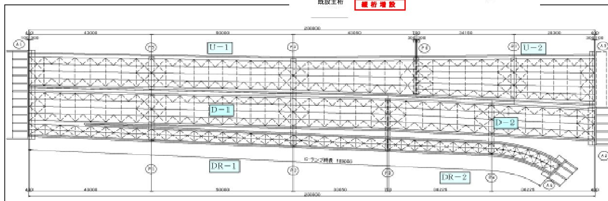
平面図及び補修概要図
