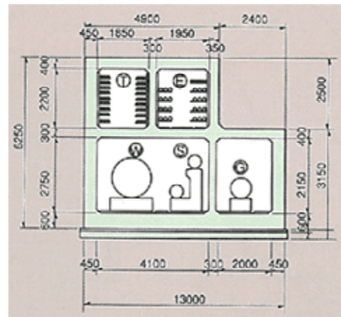
【断面図】
