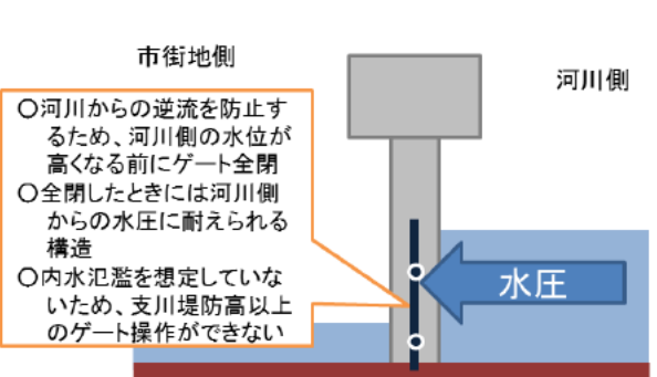
現在の樋門(イメージ)
