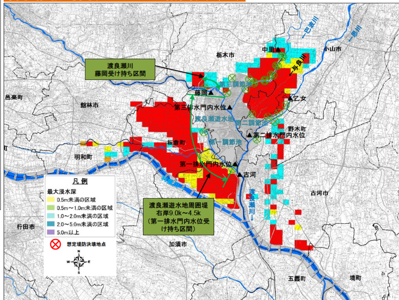
浸水継続時間(ブロック包絡図)(2/2)
