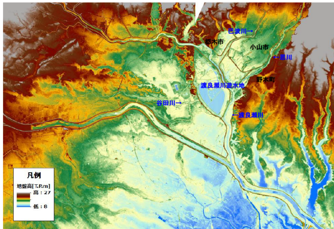
レーザプロファイルを用いた地盤高図
