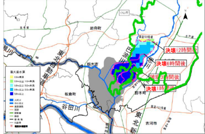
＜氾濫水到達時間図＞
