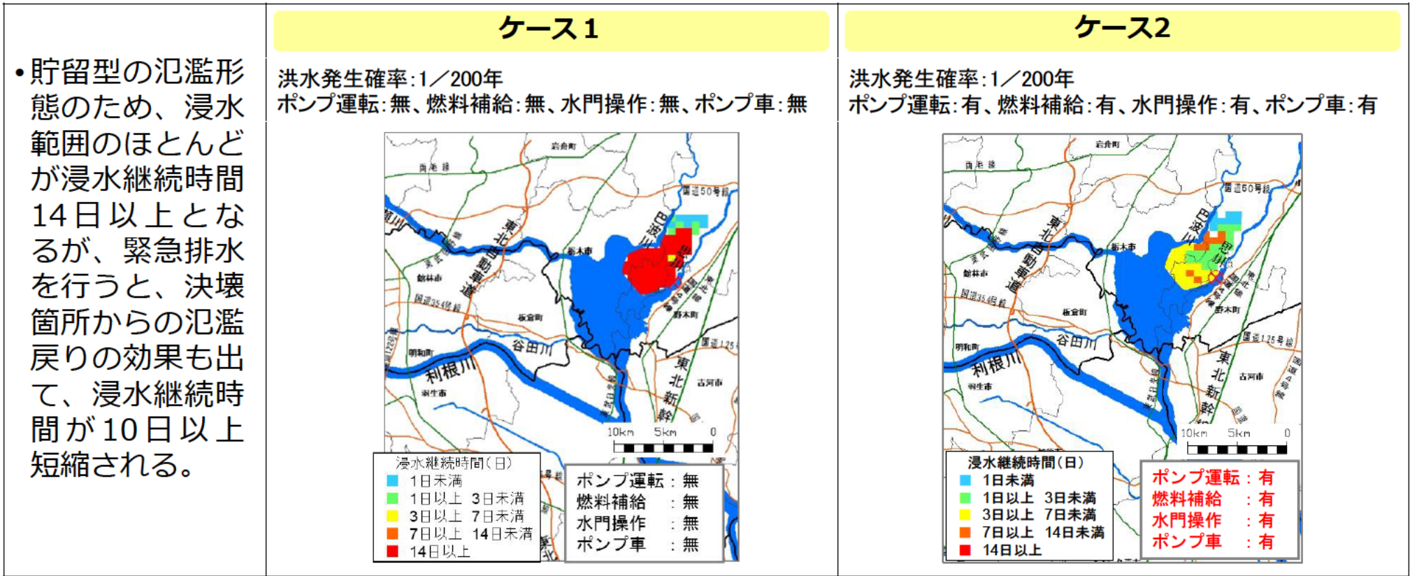
<排水対策の有無による浸水継続時間の比較> (思川右岸2.0K堤防決壊地点の浸水シミュレーション)
