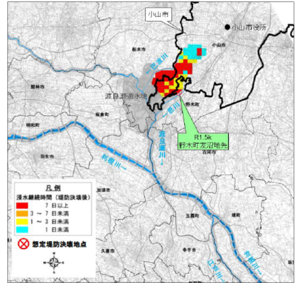
＜浸水継続時間図＞
