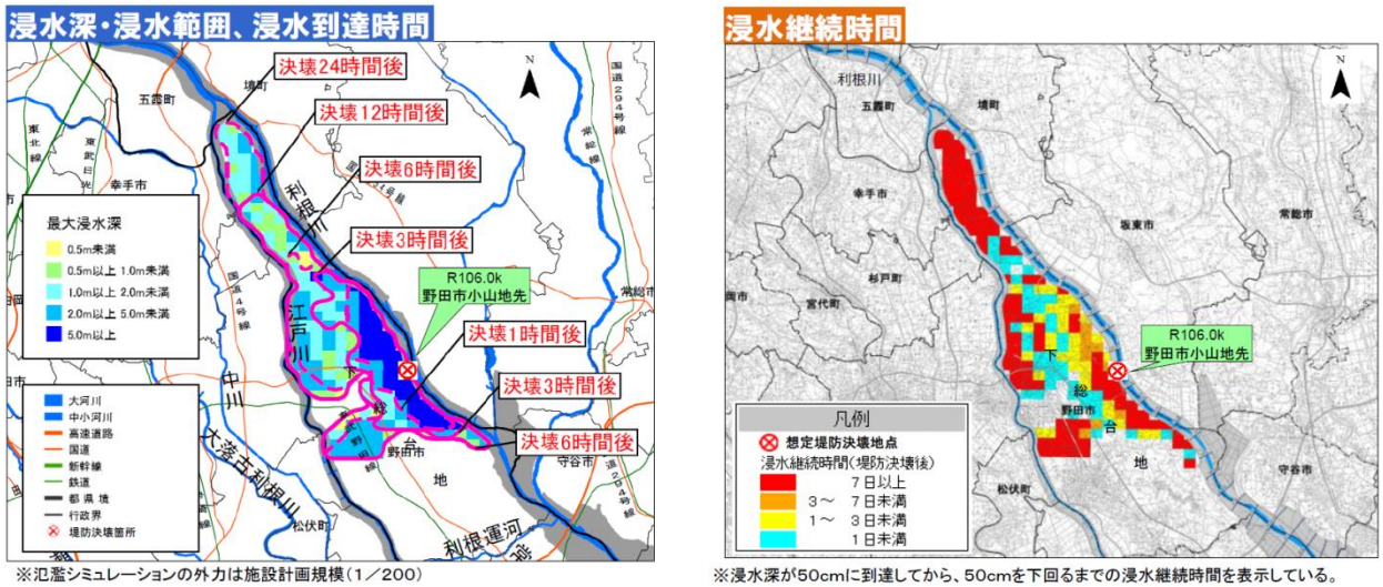
図6 浸水深・浸水範囲、浸水到達時間と浸水継続時間(利根川右岸106.0K)
