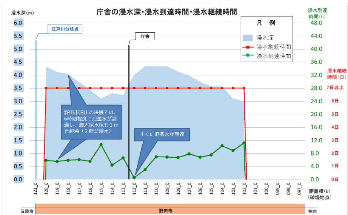
図10 浸水深・浸水到達時間・浸水継続時間(野田市役所関宿支所の例)
