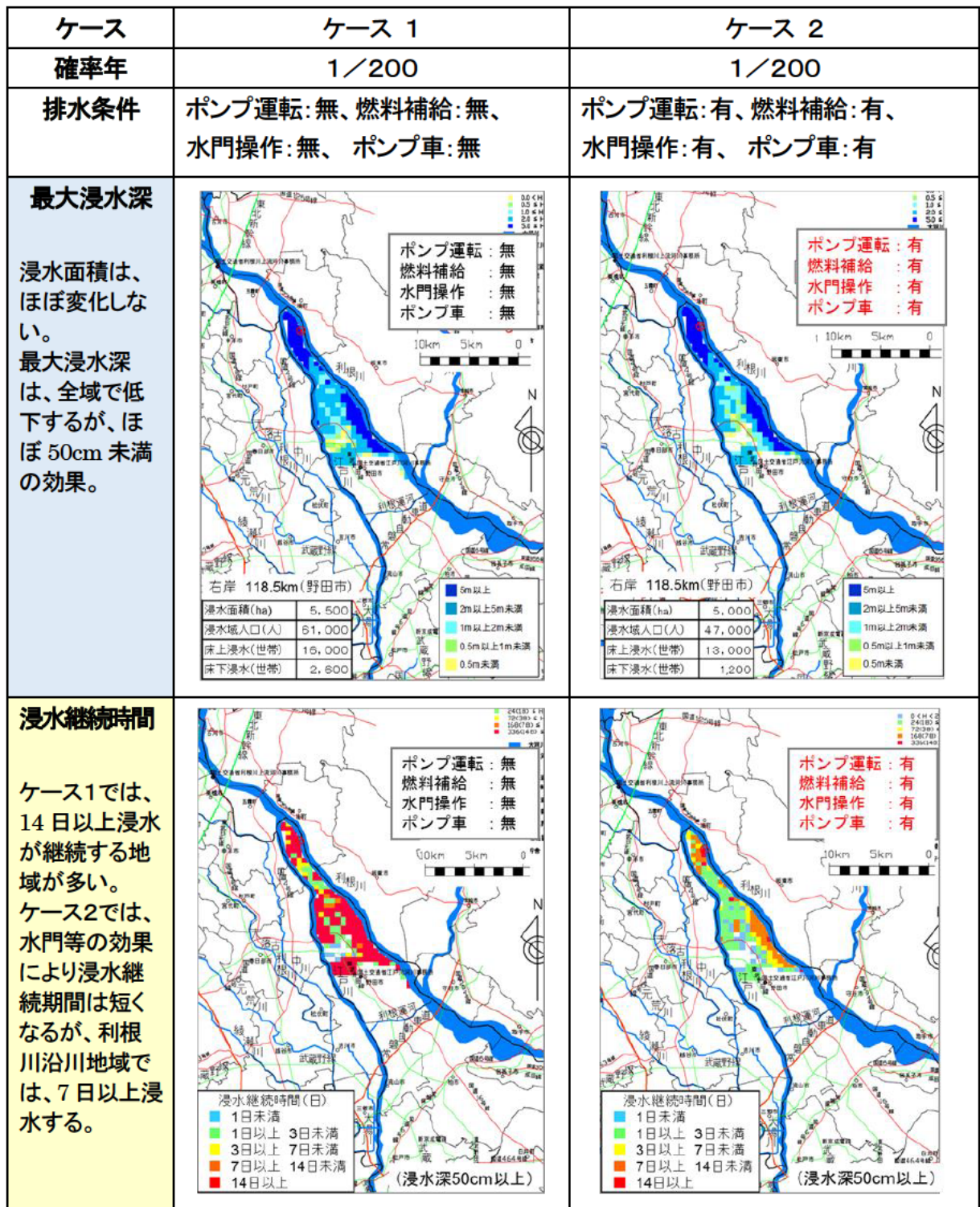
図11 排水対策の有無による最大浸水深と浸水継続時間の比較 (利根川右岸 118.5K 堤防決壊地点の浸水シミュレーション)
