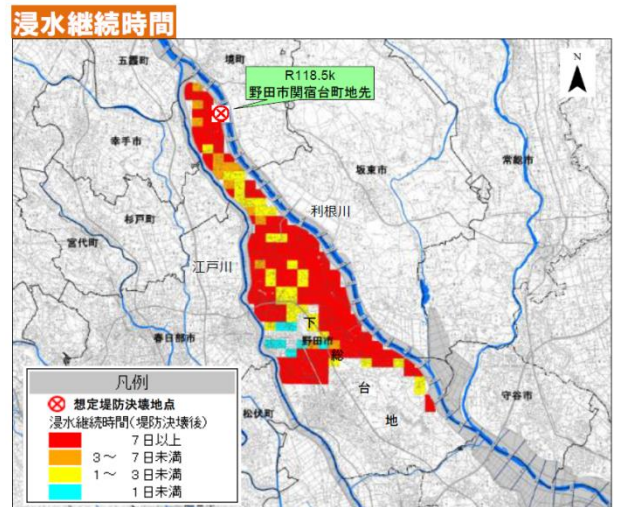
図5 浸水深・浸水範囲、浸水到達時間と浸水継続時間(利根川右岸118.5K)
