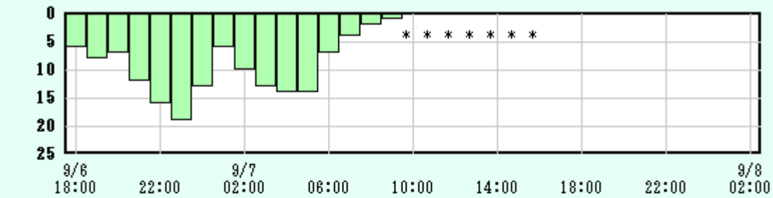
水位(m) 岩鼻水位観測所
