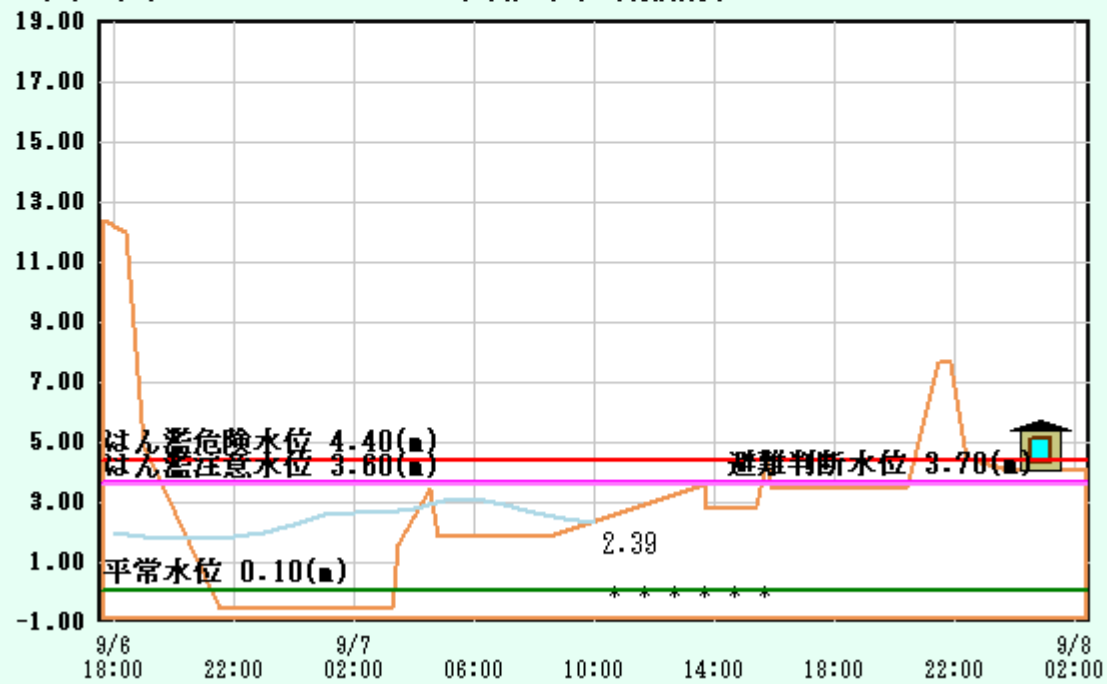
水位(m) 高松水位観測所
