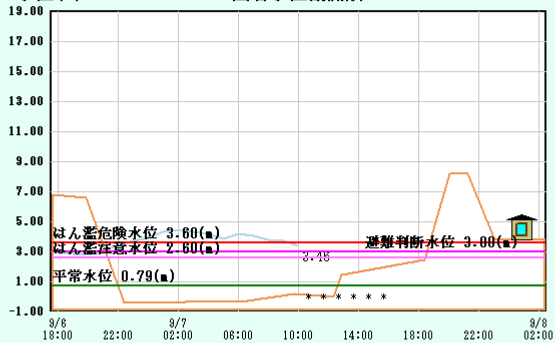
水位(m) 山名水位観測所
