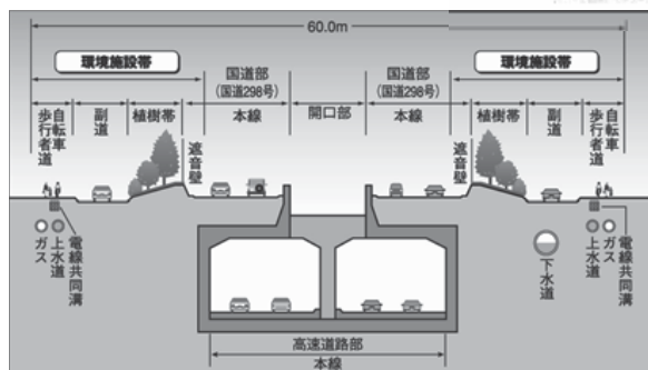
標準断面図
