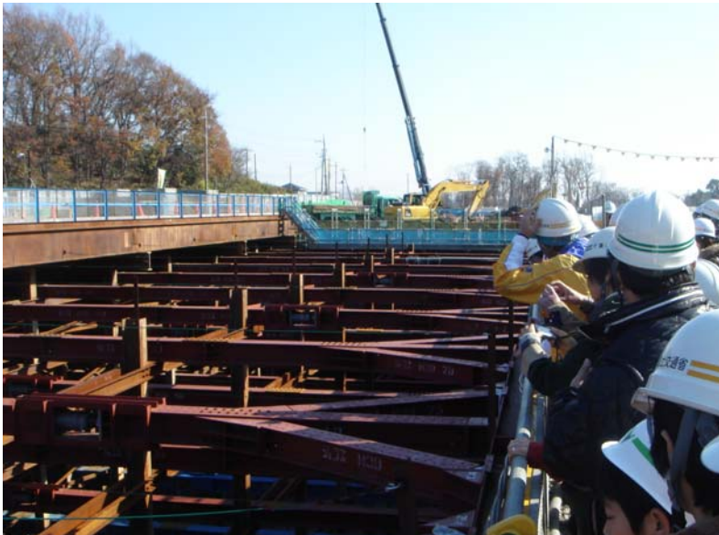
堀之内地区函渠工事
