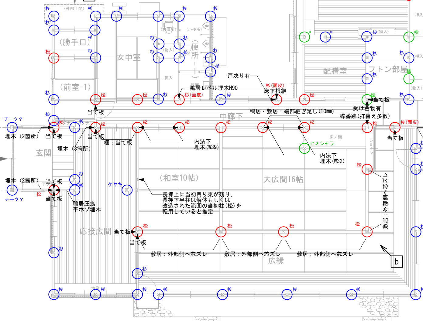
b 松正角柱が使用される和室
