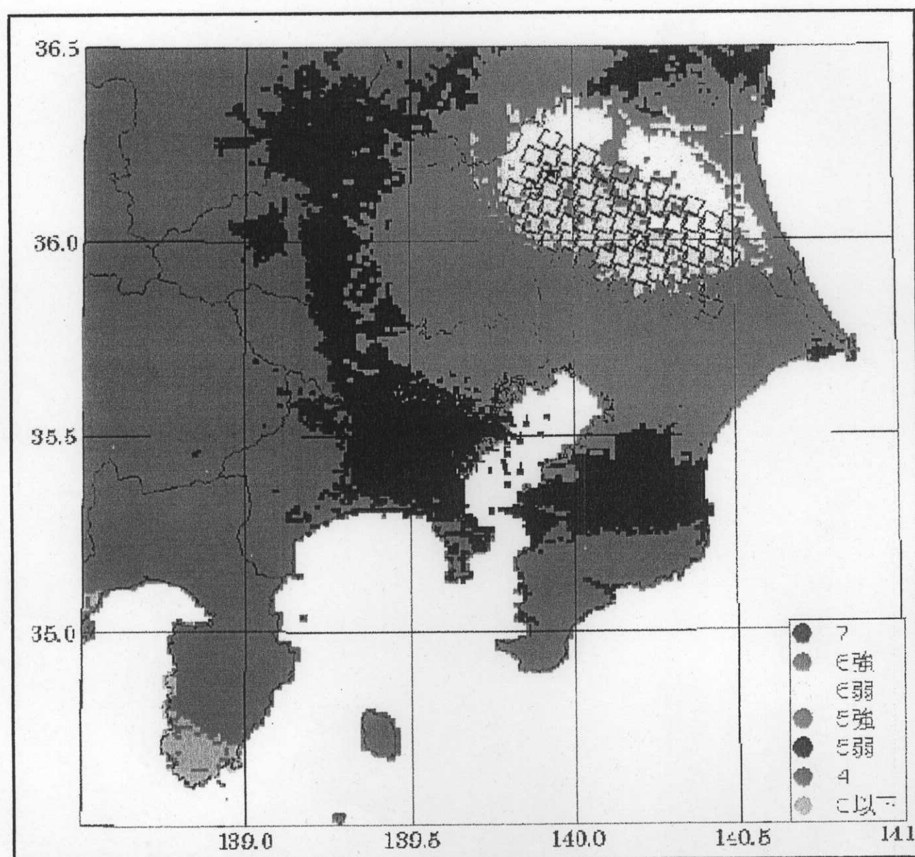
震度分布図
