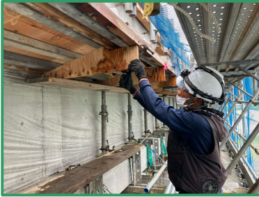
床版の型枠を解体しています。
