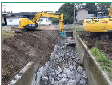
既設水路の撤去作業を行っています
