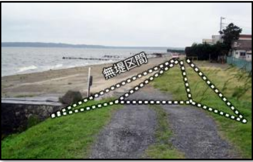
無堤部の状況(北浦右岸釜谷地区)
