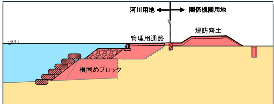
変更後の堤防構造
