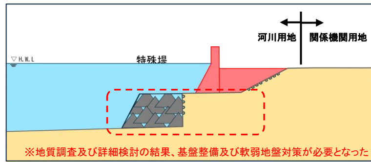
当初堤防構造
