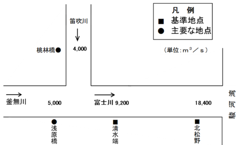
図 10 富士川流量配分図
