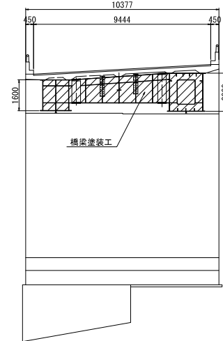
A2橋台
