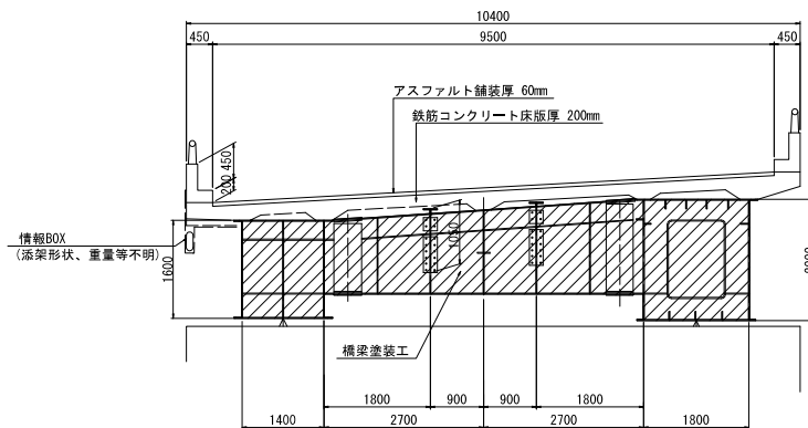
断面図 S=1:100
