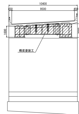
A1橋台
