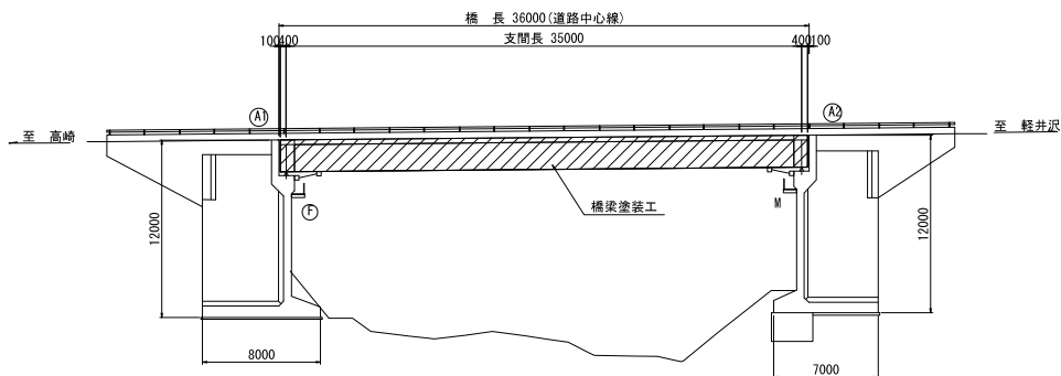
平面図 S=1:200
