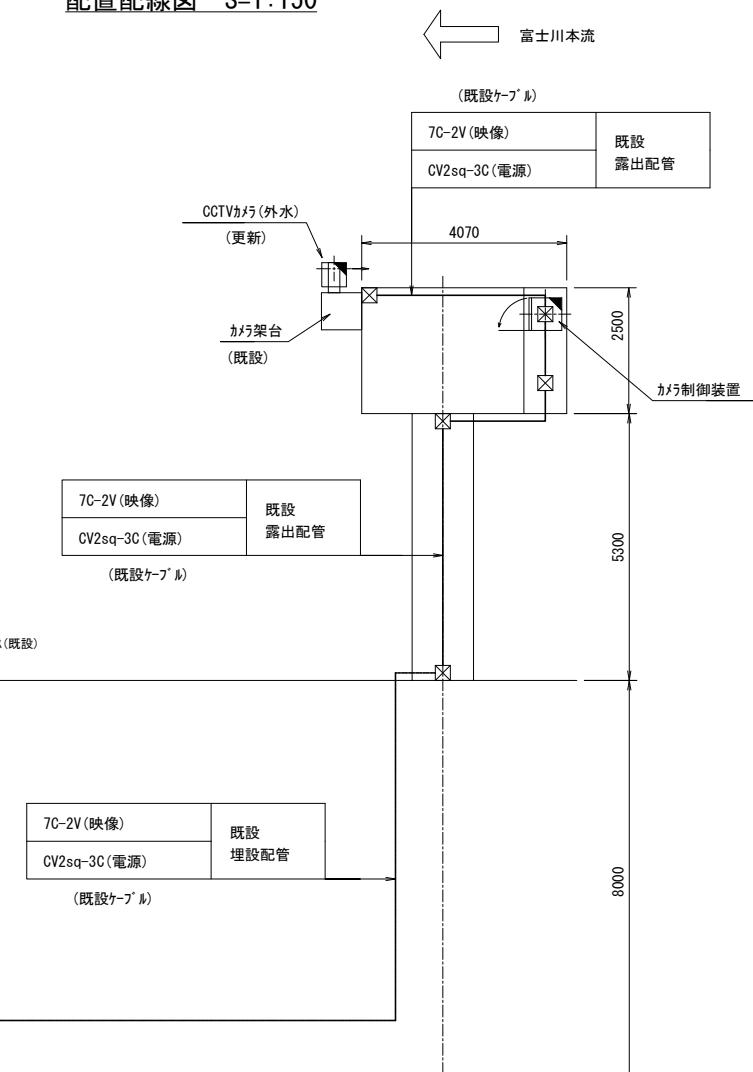
配置配線図 S=1:150
