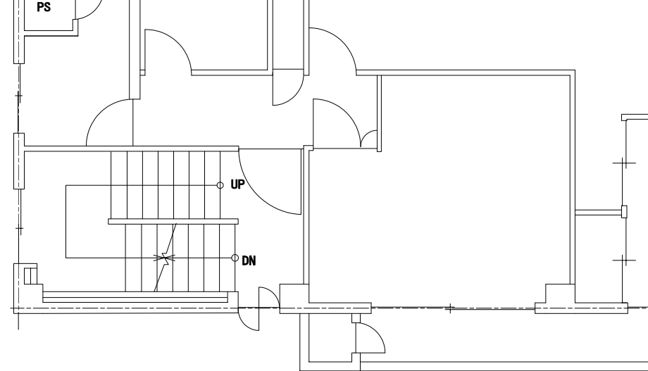
3F 平面図
