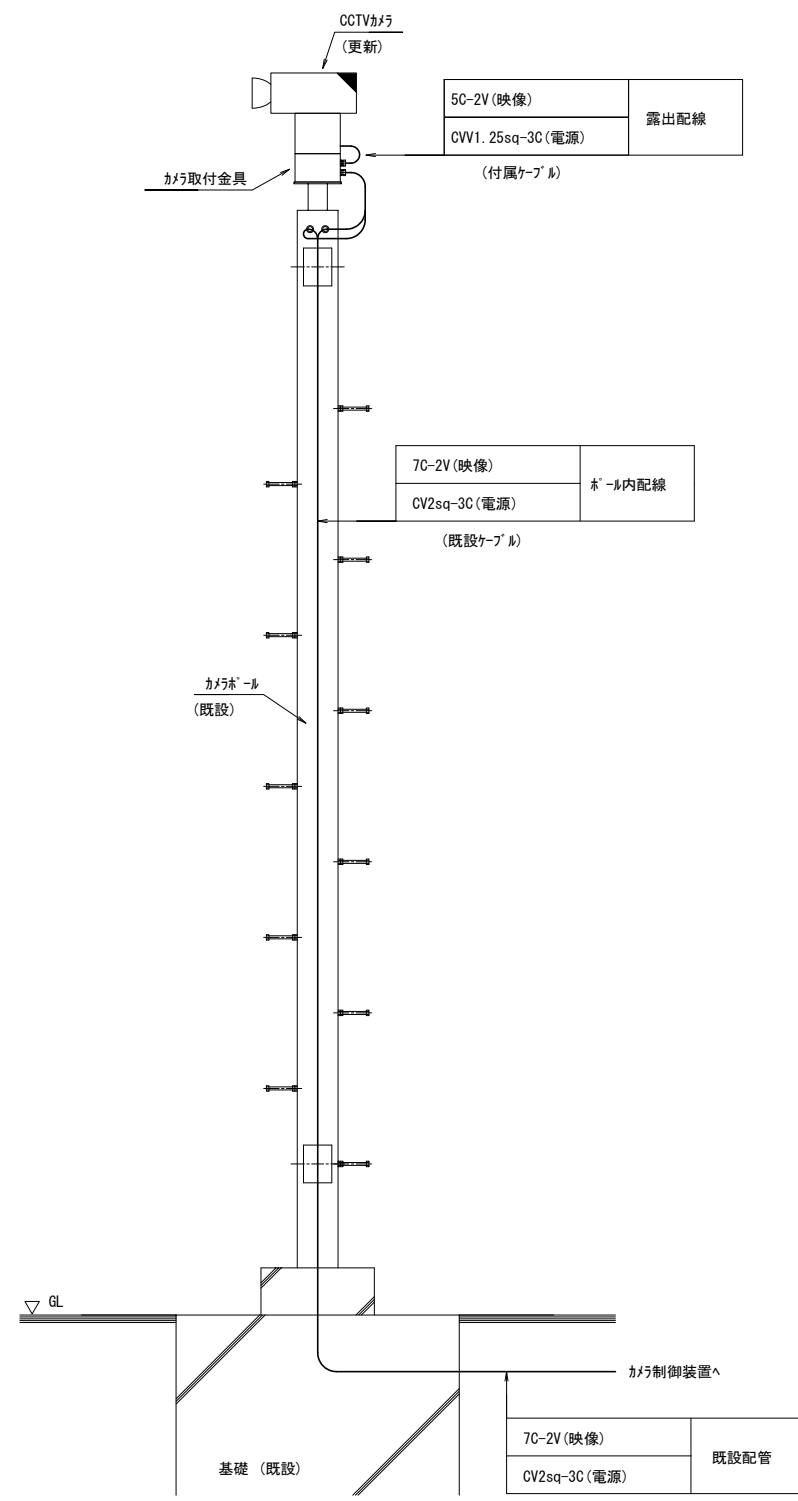
CCTVカメラ設置図 (内水) S=1:40
