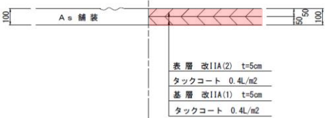
舗装構成図
