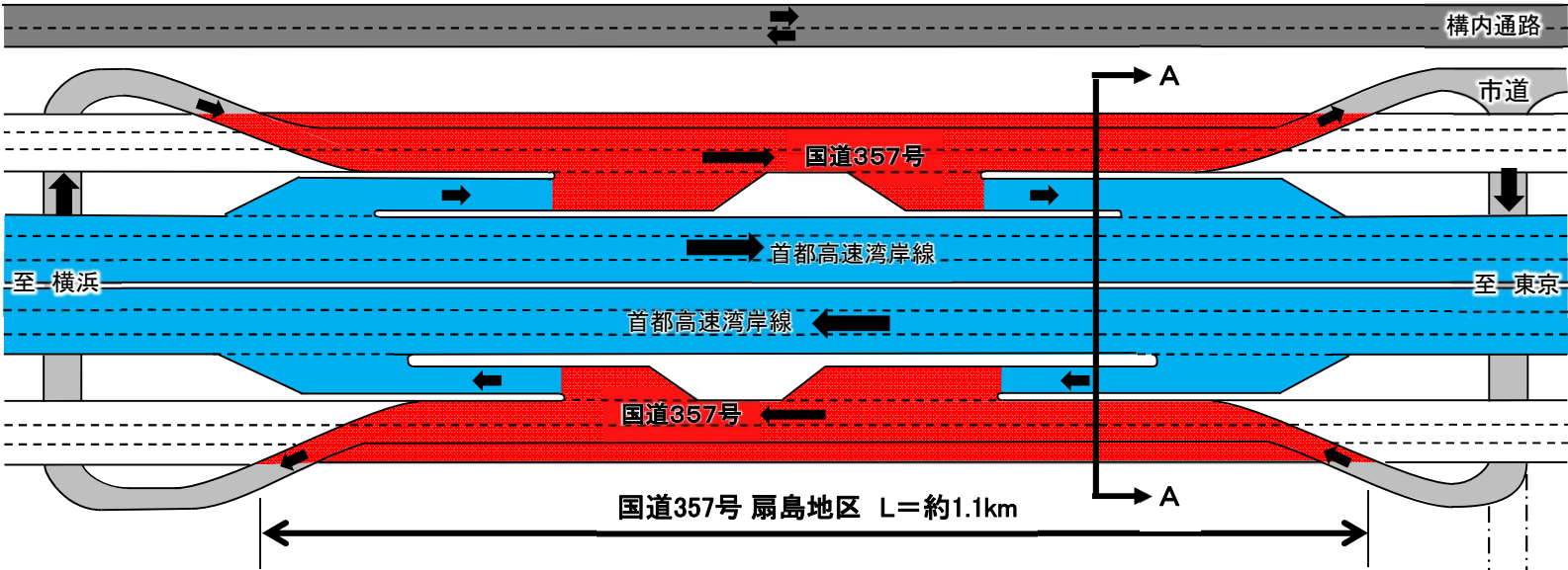
横断面図(A-A断面)
