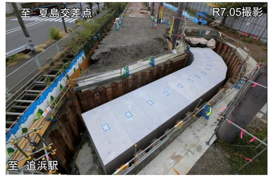
①福浦～夏島町地区の整備状況(水路移設工事)
