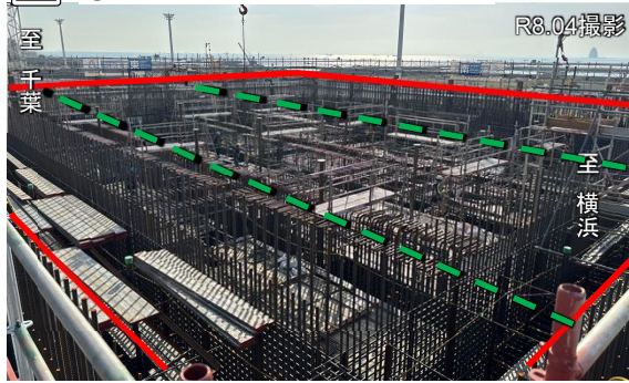
②浮島地区の整備状況(立坑鉄筋組立)
