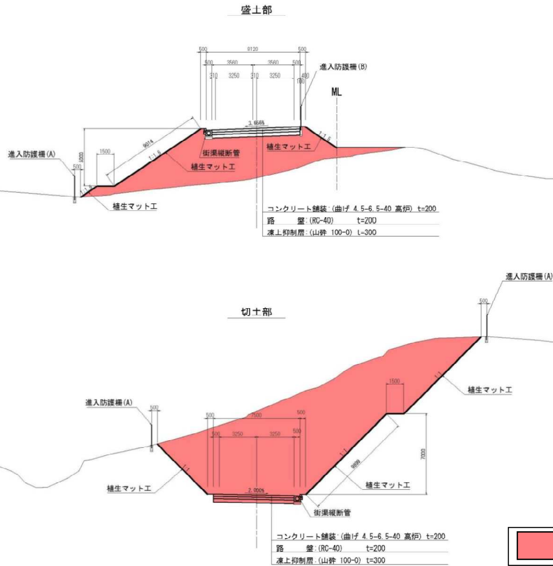
進入路標準横断面図
