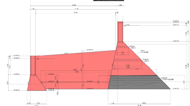
側面図
