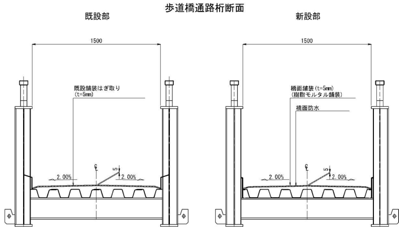
橋梁・歩道橋等補修工 S=1:15
