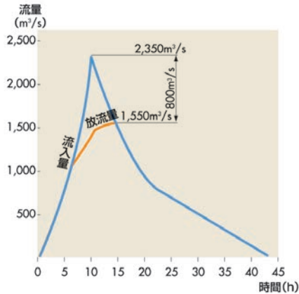
洪水調節図
