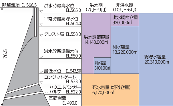
容量配分図
