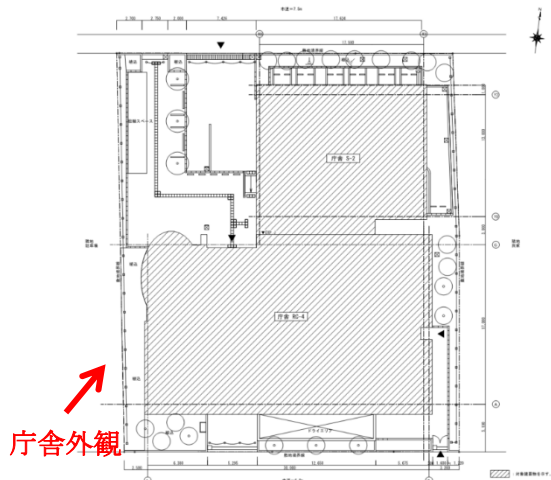
配置図
