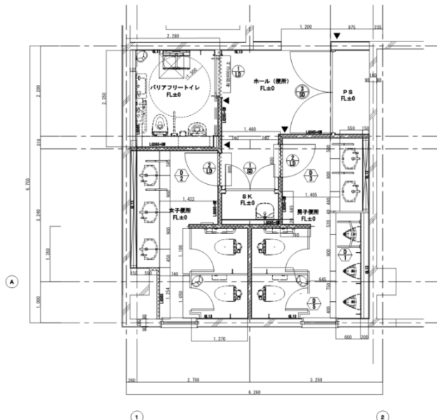
便所平面図 (改修後)
