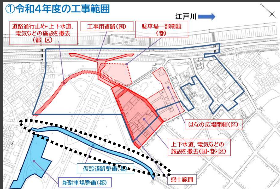
仮設道路整備後
