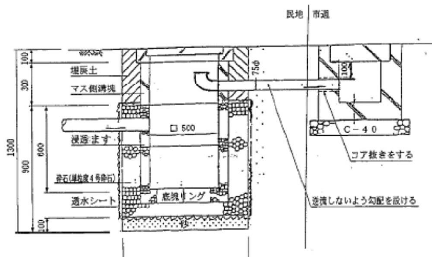
浸透枮構造図
