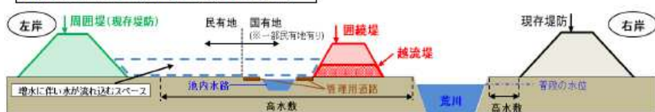
調節池の断面（上流から下流方向を見た図）
