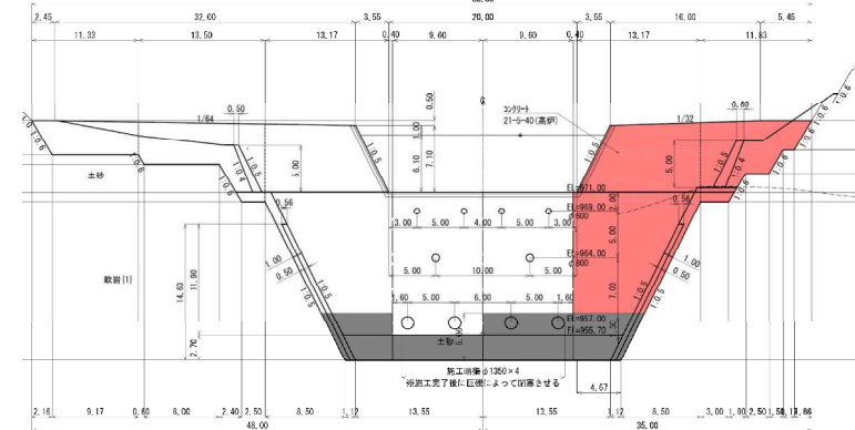
副堰堤構造図
