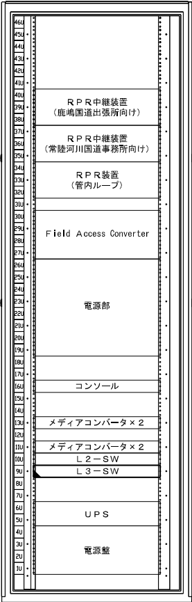
⑮光情報伝送設備架 実装図
