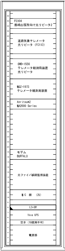
⑩光情報伝送設備架 実装図
