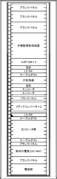
③防災系LAN收容架 実装図
