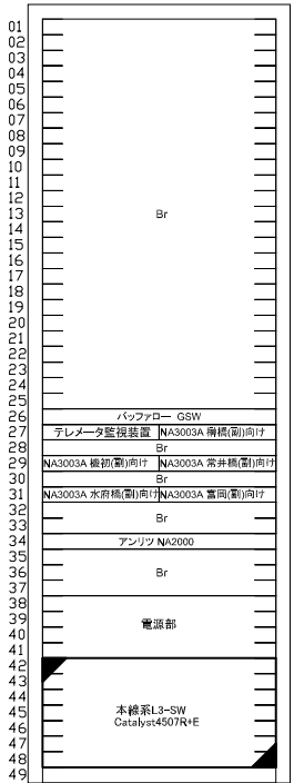
⑬L3-SW収容架 実装図
