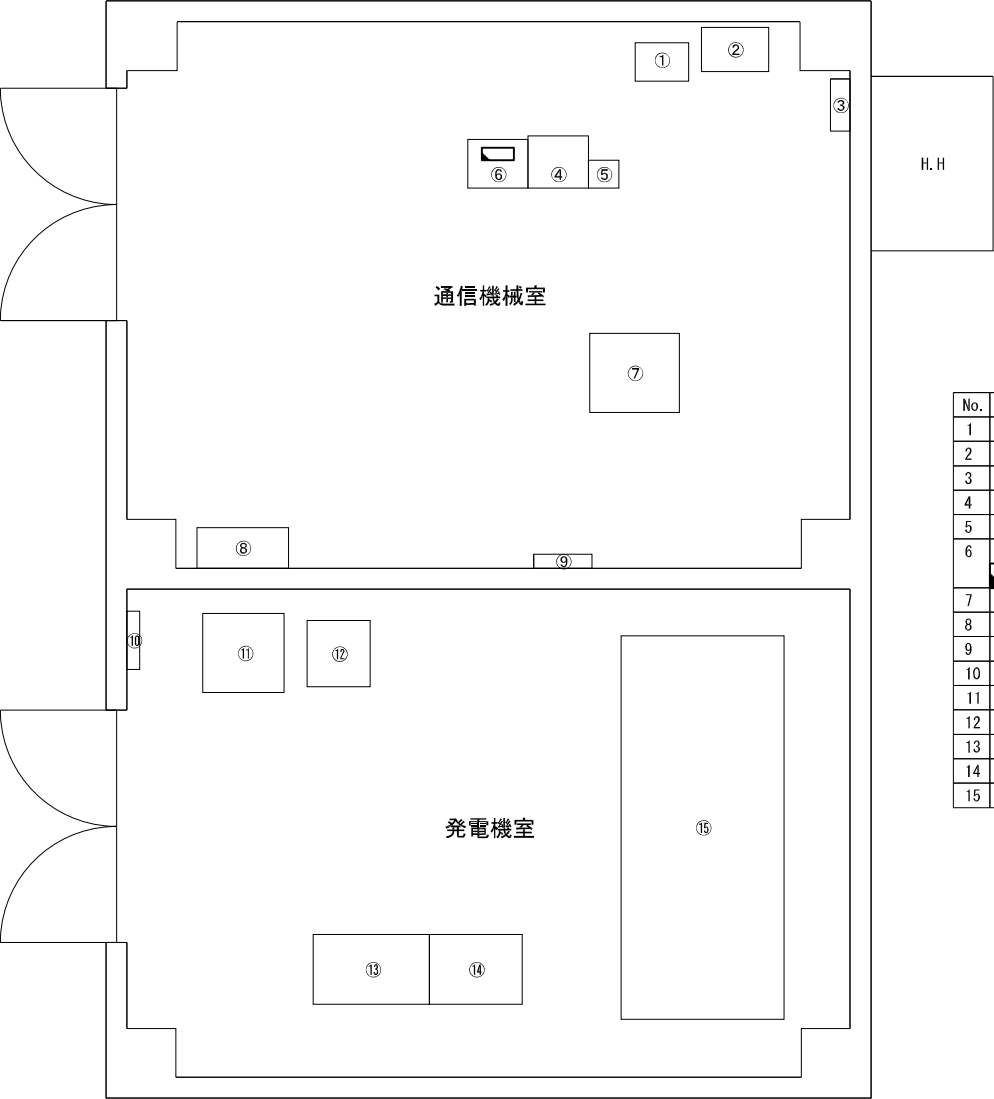
配置図
