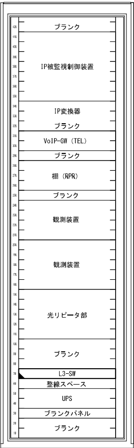
⑩L3-SW収容架 実装図
