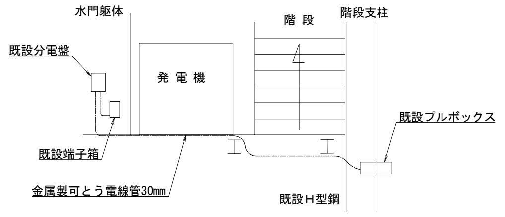
A-A' 視 配管図
