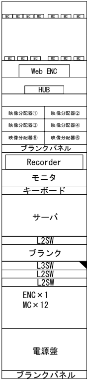
⑬ CCTV制御装置 実装図 (S=1/10)
