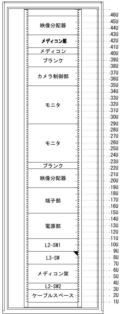
CCTV制御装置架実装図 (NS)
