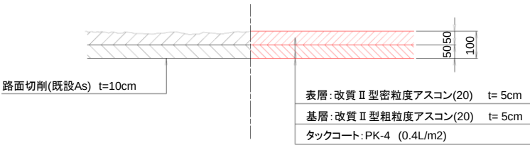
舗装構成図
