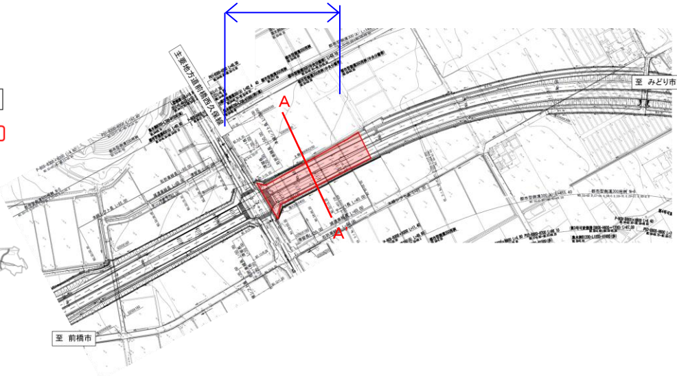
平面図
