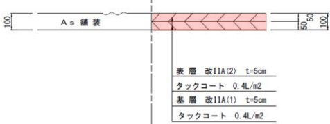
舗装構成図
