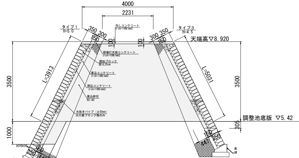
2-2 断面図 S=1:50
