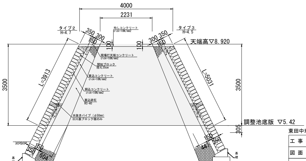
3-3 断面図 S=1:50
