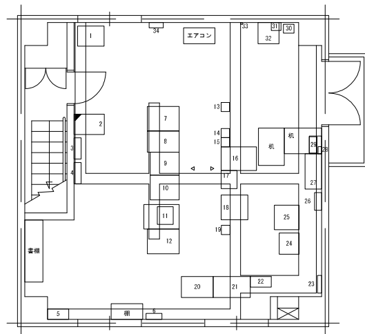
2階無線室平面図 (S=1/100) (新設)
