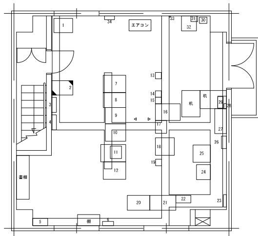
2階無線室平面図 (S=1/100) (撤去)
