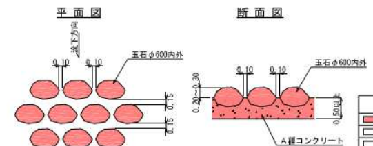
玉石張り詳細図 S=1:50
