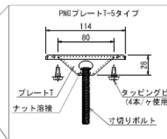
<組立用専用金具詳細図>
