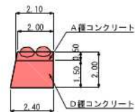
堤冠コンクリート底面詳細図 S=1:100
