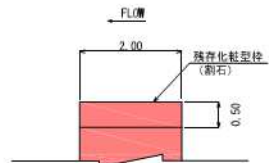
堤冠コンクリート側面詳細図 S=1:50
