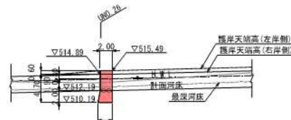
縦断面図(A-A断面) S=1:300
