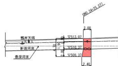
縦断面図(A-A断面) S=1:200
