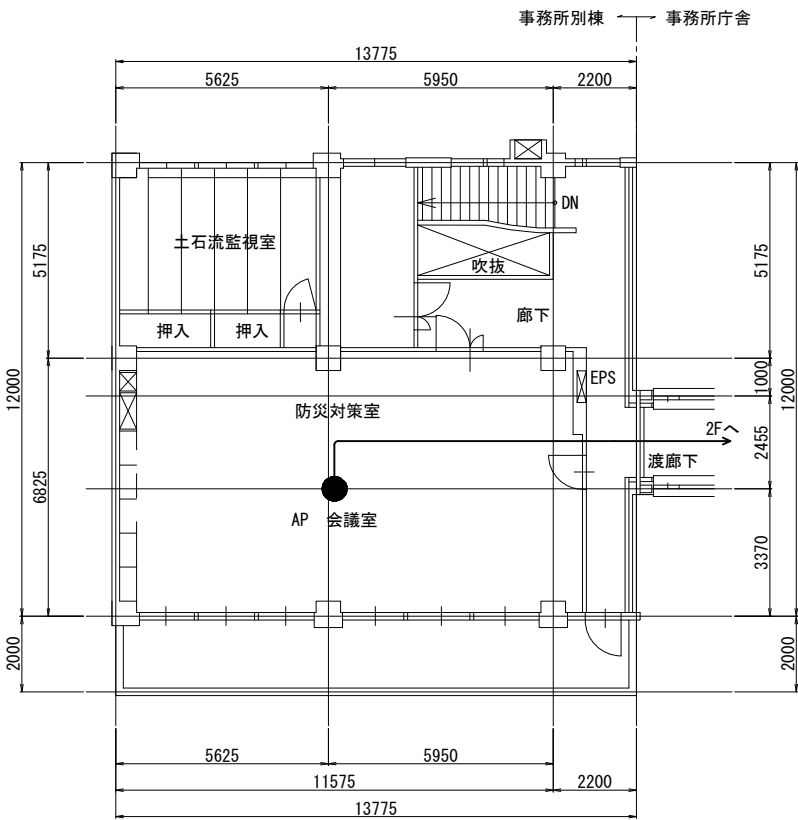
2階平面図
