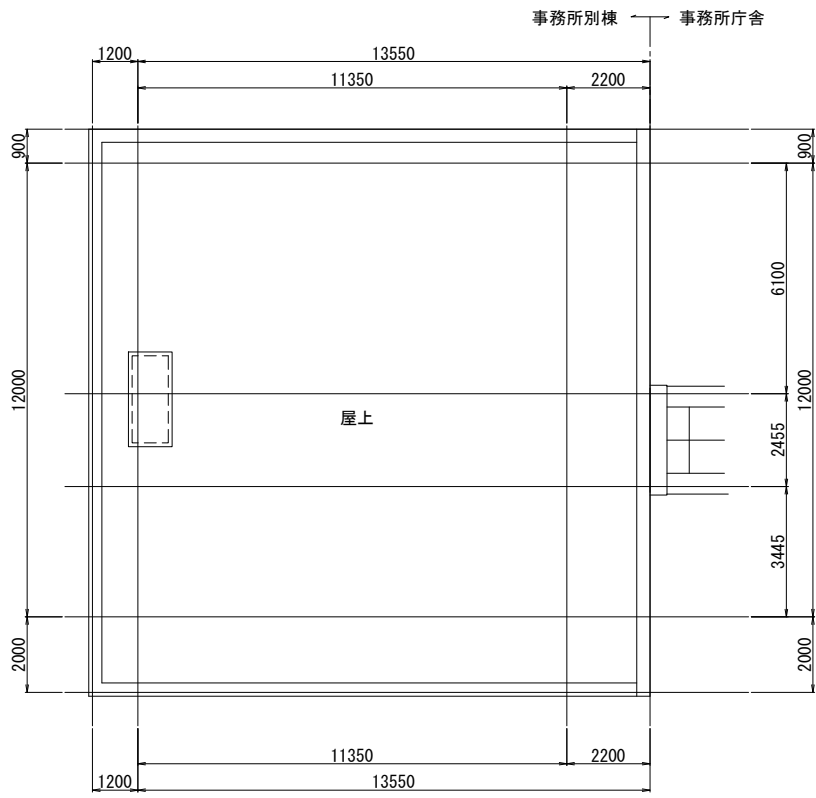
屋上平面図
