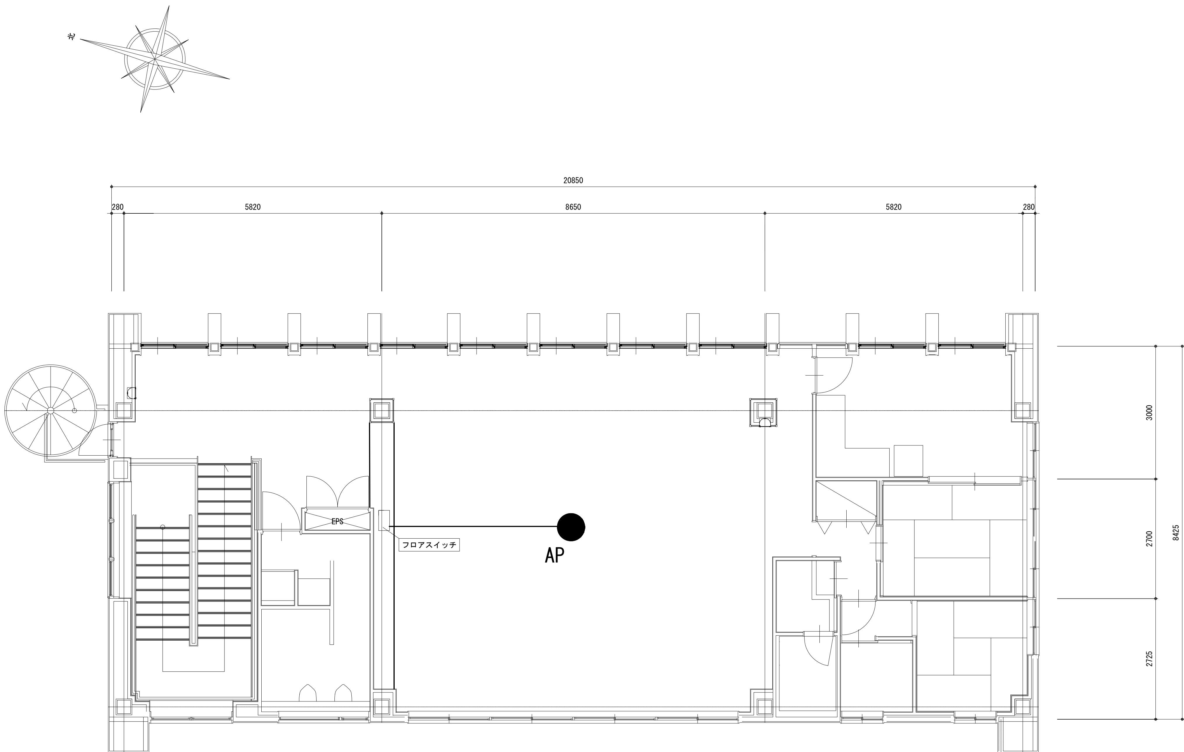
機器配置・配線図 S=1/50
