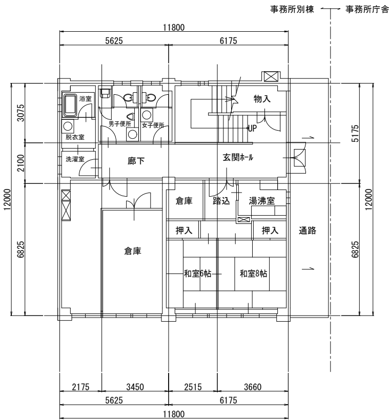
1階平面図
