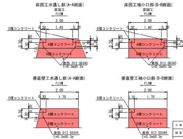
堤冠コンクリート断面図 S=1:40
