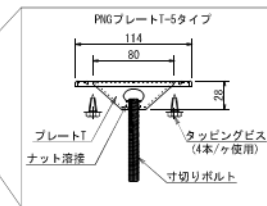
<組立用専用金具詳細図>
