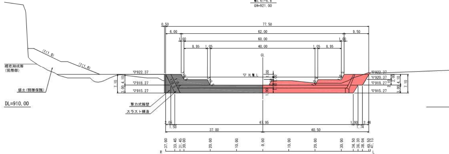
本堤正面図 S=1:300
