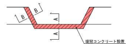
堤冠コンクリート正面模式図
