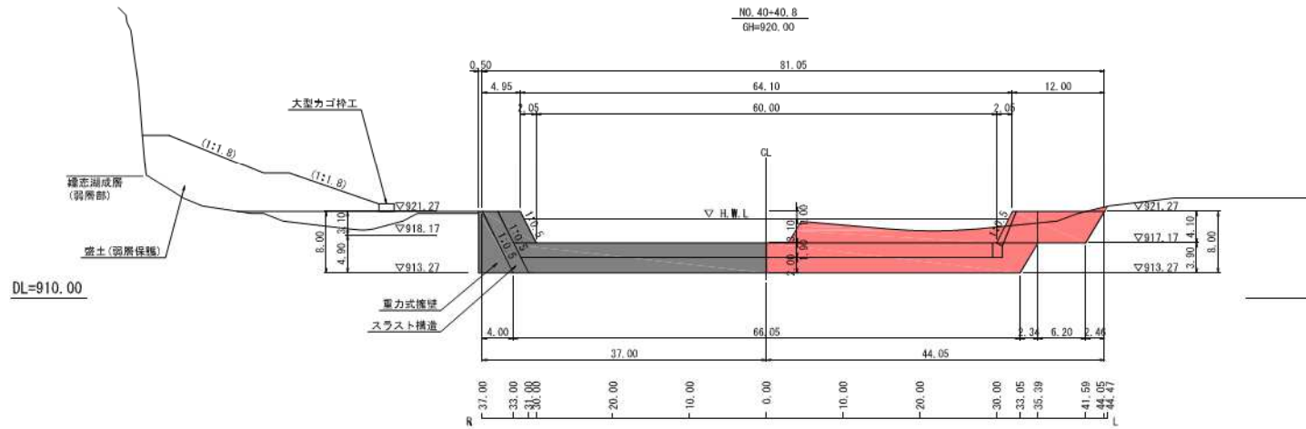
垂直壁正面図 S=1:300
