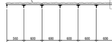
600×1200×30+40(最大断径厚) A-A断面 S=1/25
