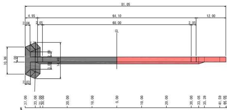
垂直壁平面図 S=1:300
