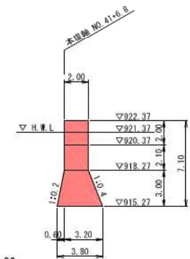
本堤断面図 S=1:150
