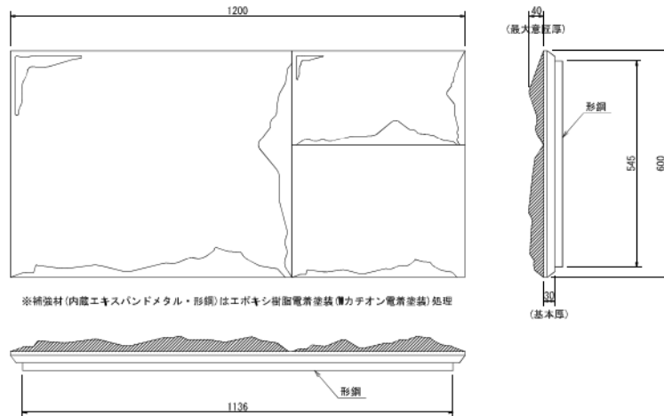
残存化粧型枠詳細図 S=1/6 ※PNメッシュ使用製品(標準打設高1.5m以下)
