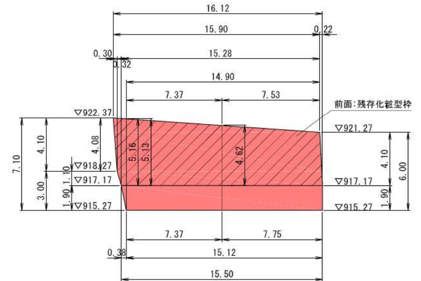
側壁工側面図 S=1:100
