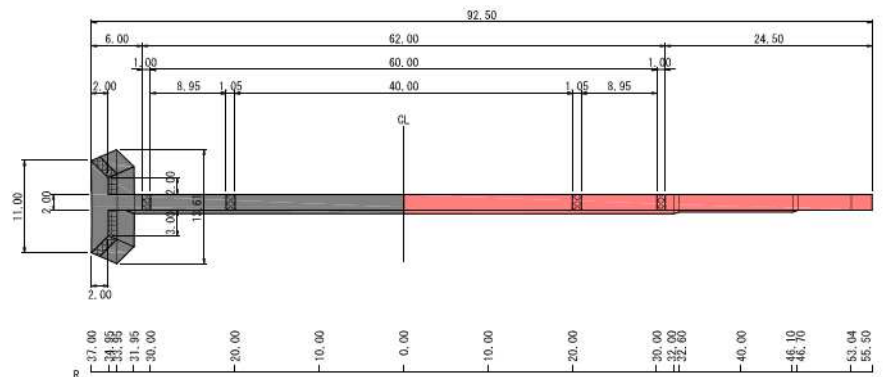
1号帯工平面図 S=1:300
