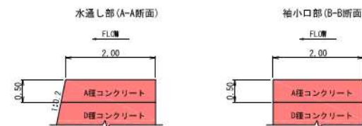
堤冠コンクリート断面図 S=1:40
