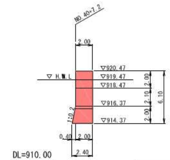
1号帯工断面図 S=1:150
