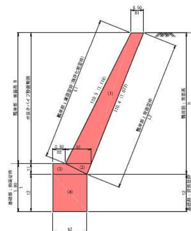
側壁工模式図 S=1:50
