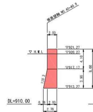
垂直壁断面図 S=1:150
