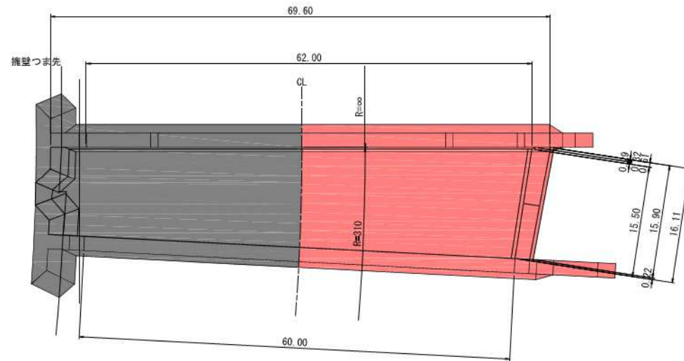
平面図 S=1:250
