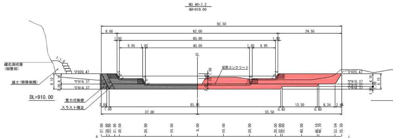
1号帯工正面図 S=1:300
