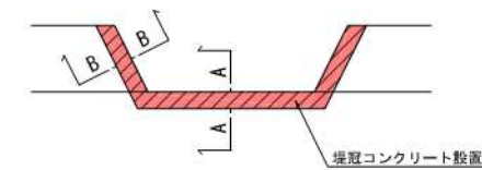
堤冠コンクリート断面図 S=1:40
