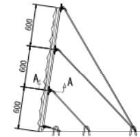
<組立用専用金具詳細図>
