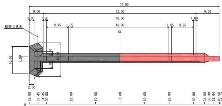
本堤平面図 S=1:300
