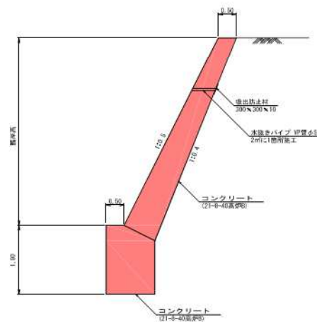
側壁工標準断面図 S=1:50
