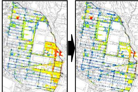
浸水シミュレーションによる対策効果検証
