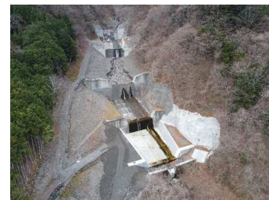
池の沢第二砂防堰堤工事(R7年度完成)
