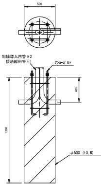
照明灯基礎詳細図
