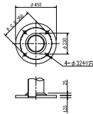
照明灯基礎詳細図
