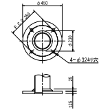
照明灯基礎詳細図
