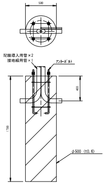
照明灯基礎詳細図
