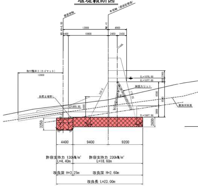
堰堤縦断面図
