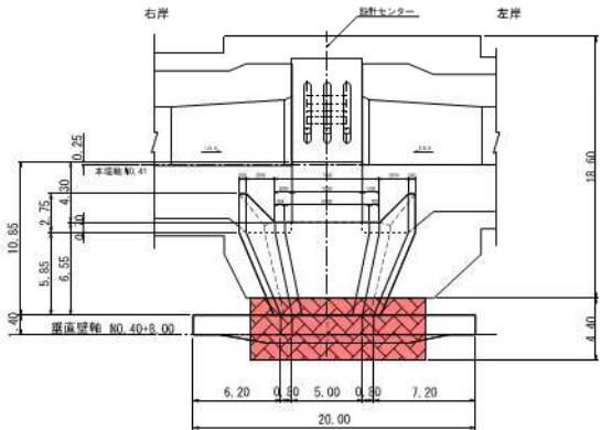
垂直壁平面図
