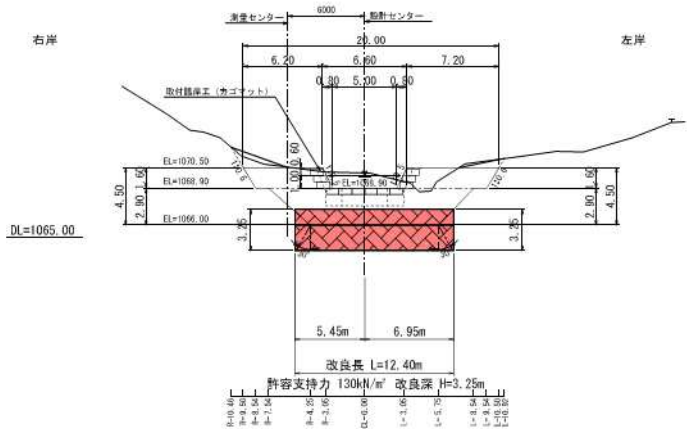
垂直壁正面図
