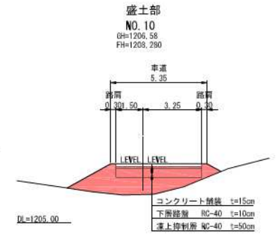
管理用道路 1 標準断面図 S=1:100
