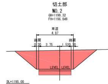
管理用道路 1 標準断面図 S=1:100
