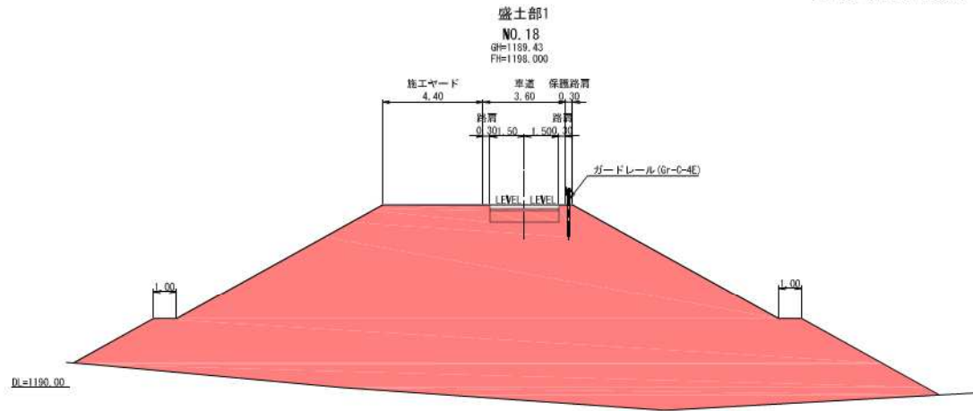
工事用道路 1 標準断面図 S=1:100
