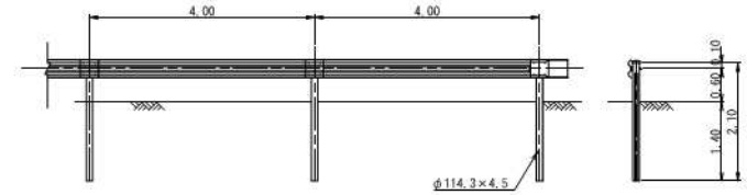
ガードレール (Gr-C-4E) S=1:50
