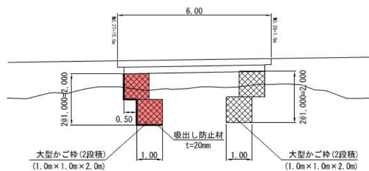
断面図 S=1:250
