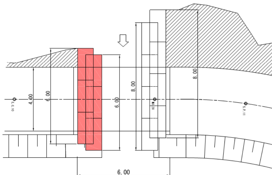
平面図 S=1:250
