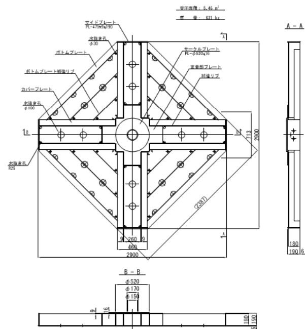
鋼製受圧板構造図
