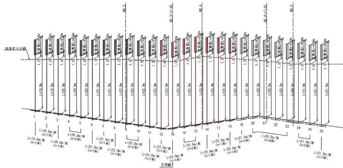
L3 展開図 S=1:200
