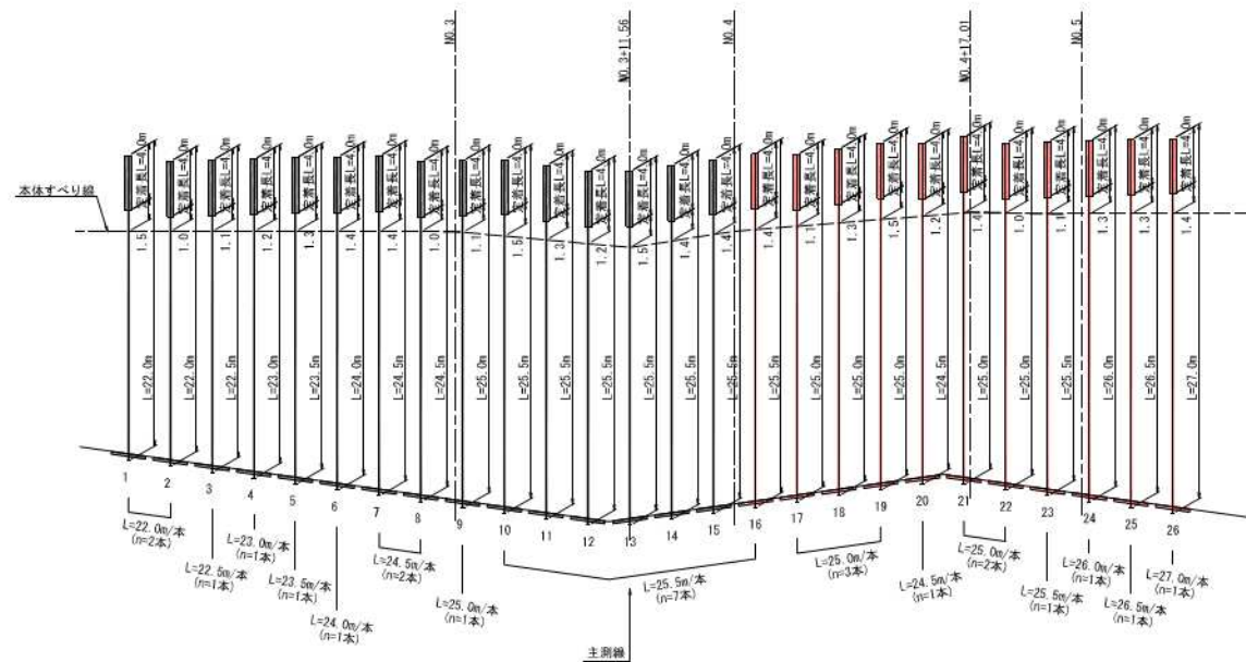
L5 展開図 S=1:200
