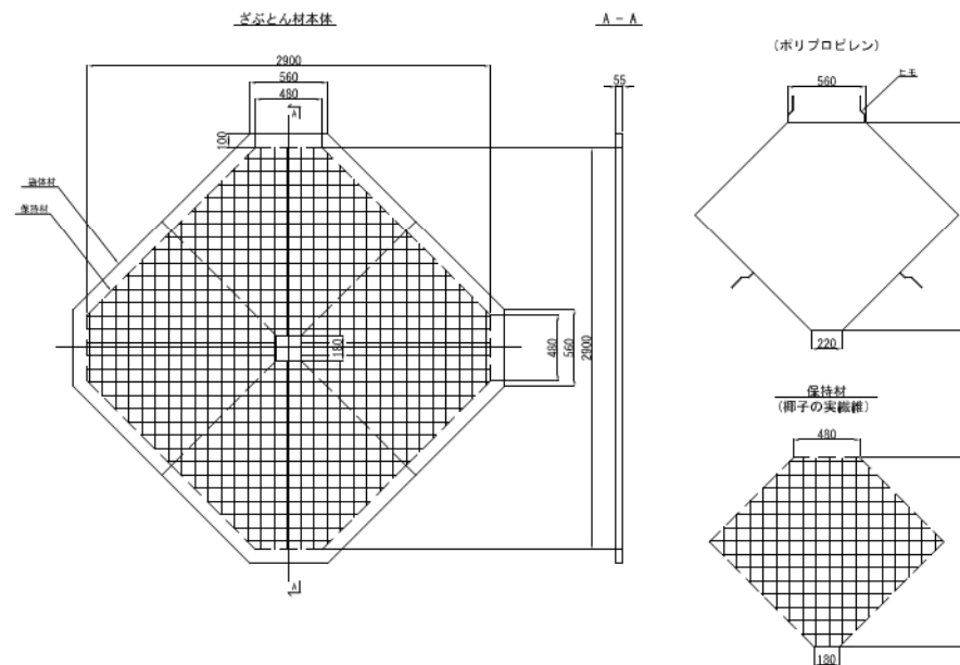
ざぶとん材構造図
