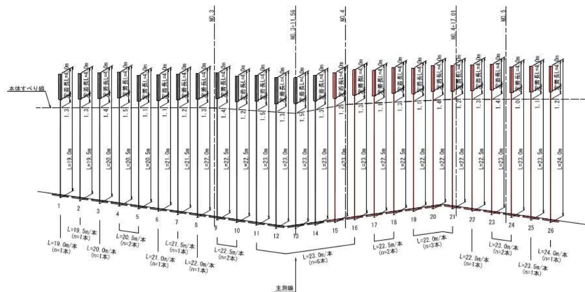
L5 展開図 S=1:200
