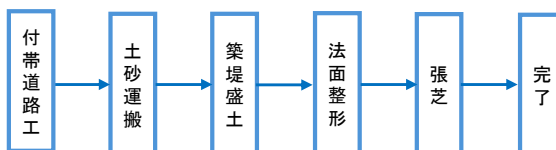
三反田地区施工フロー
