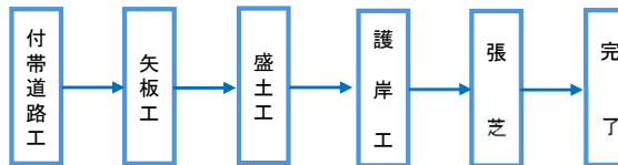
美田多町・関戸地区施工フロー
