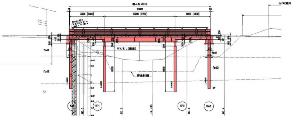
仮橋一般図
