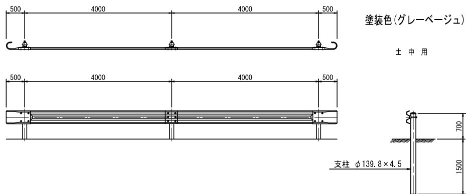
ガードレール (Gr-A-4E)
