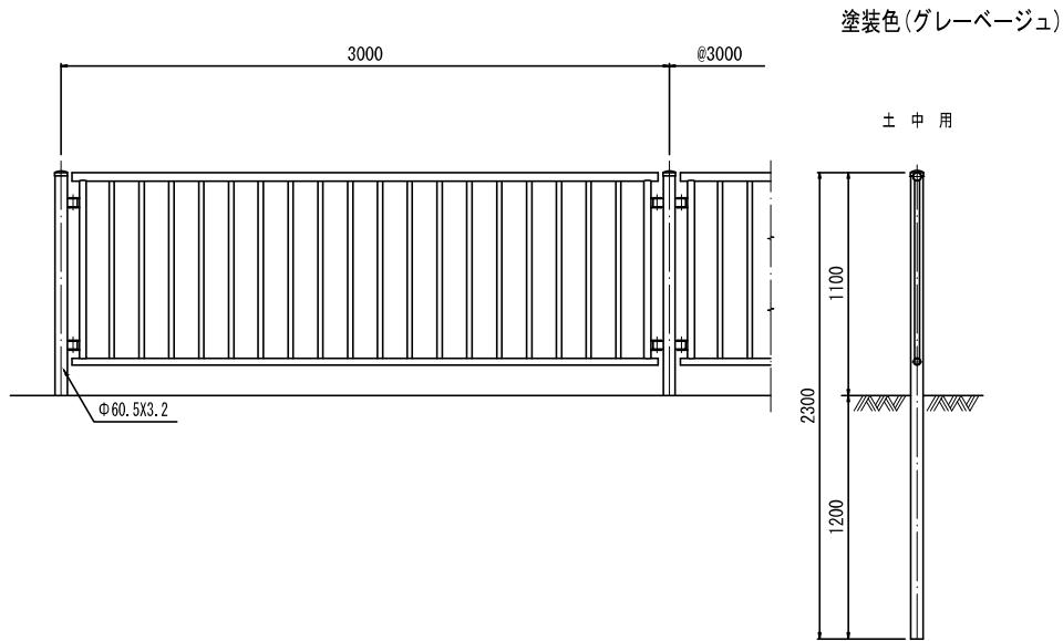
ガードパイプ (Gp-Bp-2E)
