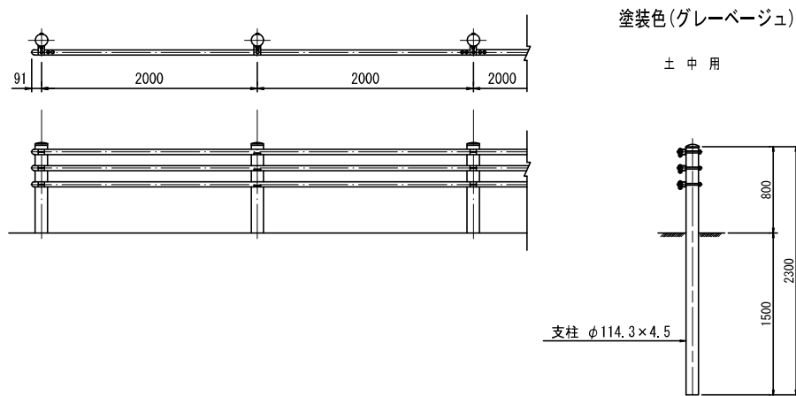
ガードパイプ (Gp-Bp-2E)
