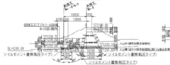
越流部側面図
