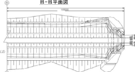
B-B 平面图
