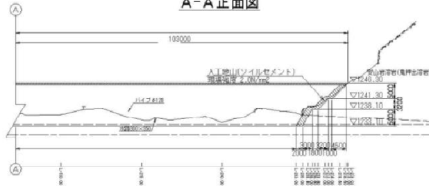
A-A 正面图
