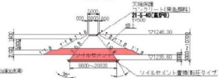
非越流部側面図 右岸側
