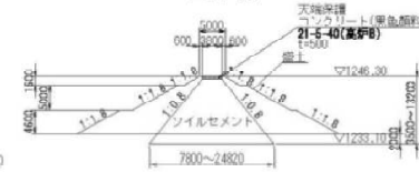
非越流部側面図 左岸側
