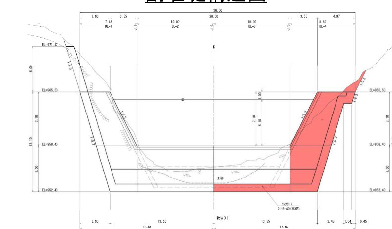
側面図
